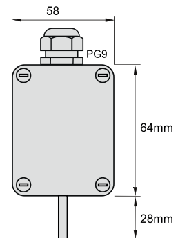
fig. 1. Dimensions (mm)
