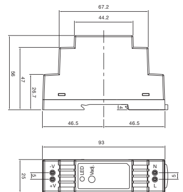
fig. 1. Dimensions (mm)
